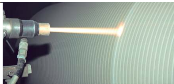
Torche projection revêtement sur rouleau immergé
