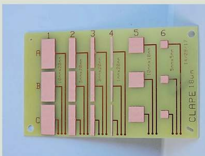
Photo d'un PCB revêtu de cuivre par Cold Spray
